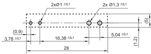
垂直安装型
