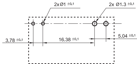
水平安装型
